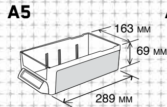
A5 A5 Cabinet Drawer
